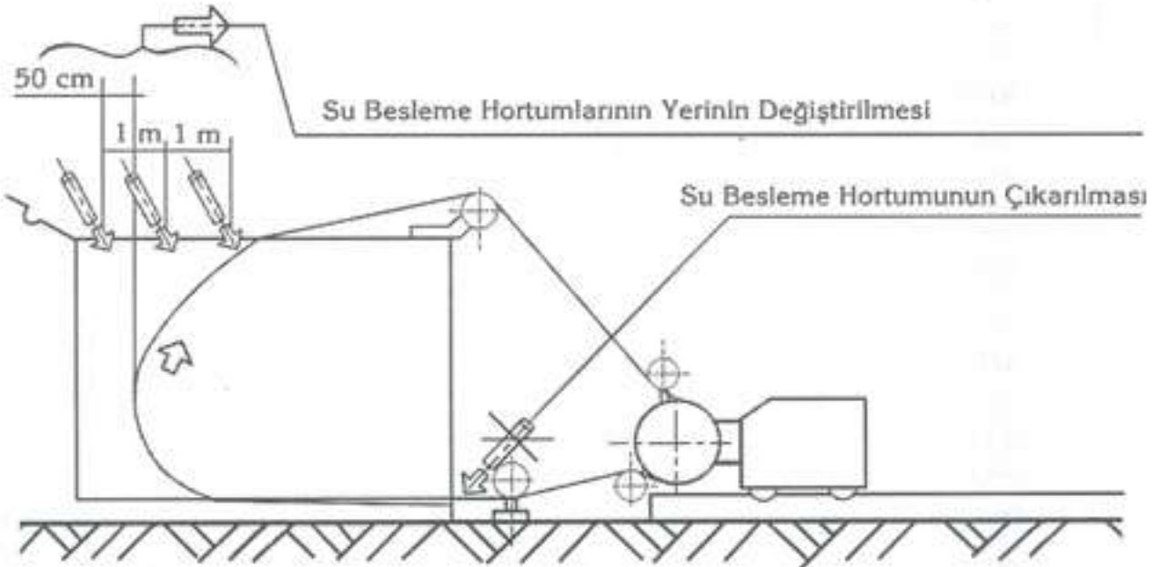
Şekil 26. B Soğutma Sisteminin Modifikasyonu
